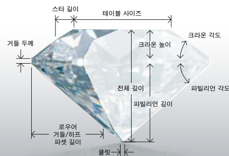
다이아몬드의 구조
